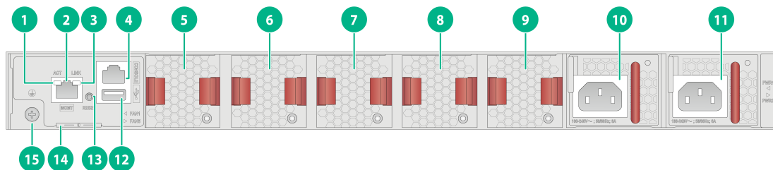
图2-2 S9600XP-32H-G 后面板示意图
